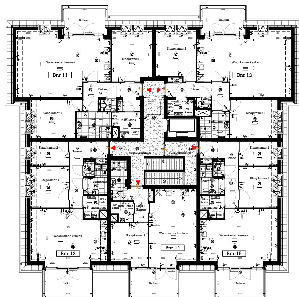
PLATTEGROND TWEEDE VERDIEPING
