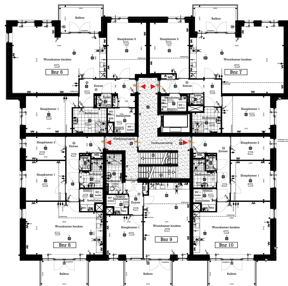
PLATTEGROND EERSTE VERDIEPING
